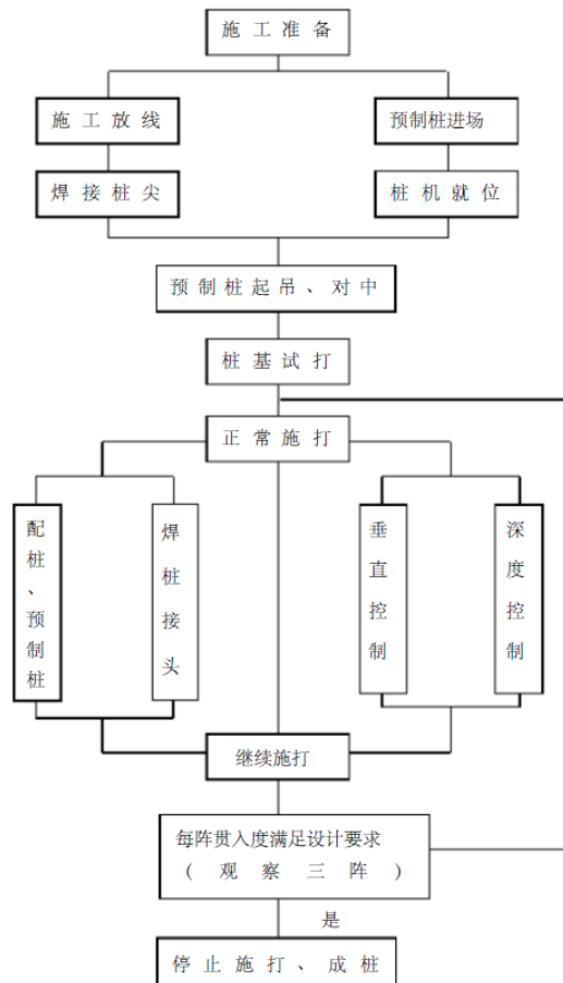
图 2-4 锤击预制桩工艺流程图
