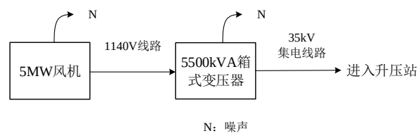
图 4-1 建设项目运营期产污节点
