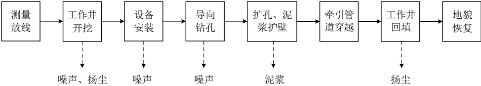
图 2-8 拉管施工产污节点图
